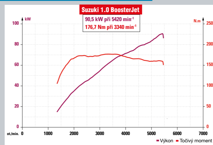
Absolutní naměřené hodnoty nejsou nic moc, ale průběh točivého momentu vyhoví jak defenzivním, tak aktivnějším řidičům. Jediné suzuki za něj dostává jedničku i proto, že křivky jsou plynulé bez houpání.
